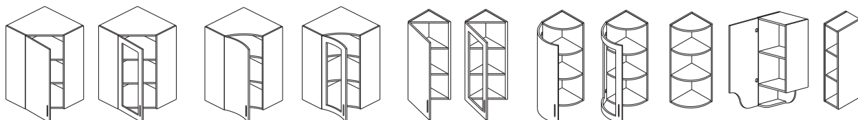
B201-60 (Л/П) BB201-60 (Л/П) B202-60 (Л/П) BB202-60 (Л/П) B203-30 BB203-30 B204-32 BB204-32 B205-30 B206-30(Л/П) B208-15 60 x 60 см 60 x 60 см 60 x 60 см 60 x 60 см (Л/П) (Л/П) (Л/П) (Л/П) B205-22 B206-40(Л/П) B208-20
