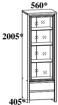
Шкаф REG1W2S
